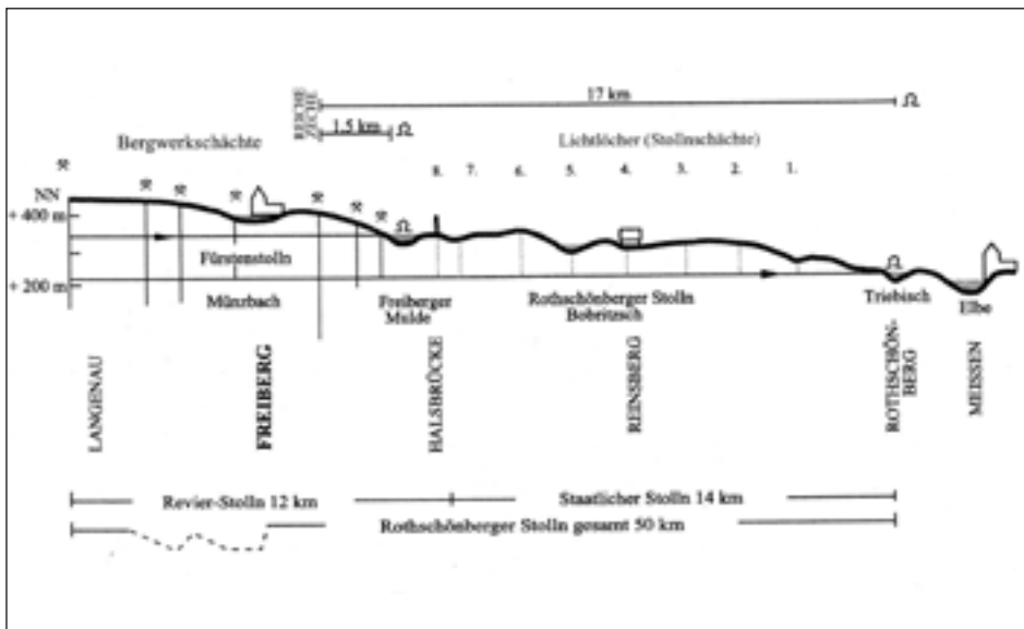
Abb. 10: Schematischer Schnitt durch den Rothschönberger Stollen, bei dessen Bau (1844–1877) durch Professor Julius Weisbach die «Neue Markscheidekunst» eingeführt wurde, Zeichnung H. Pforr.
