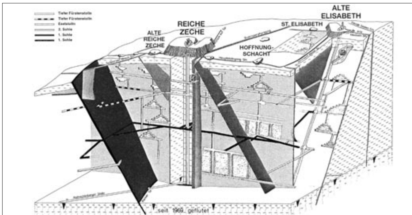
Abb. 3a: Räumliches Bild der «Himmelfahrt Fundgrube» mit Erzgängen, Schächten und den Stollen (Fürstestolln und Roths Schönberger Stolln).
