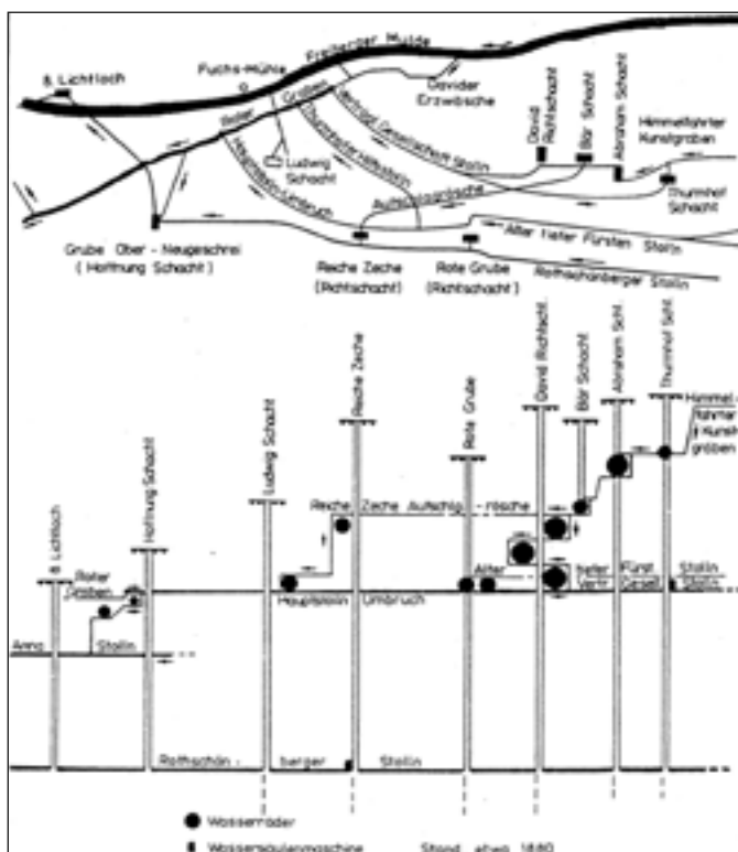
Abb. 4: Kaskadenartige Nutzung der Fallhöhe für wasserbetriebene Kraftmaschinen (Wasserräder, Kolbenkraftmaschinen) in der «Himmelfahrt Fundgrube», Zeichnung H. Pforr.
