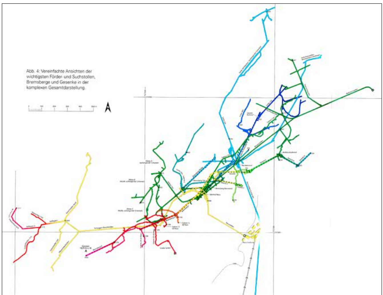
Vereinfachte Ansicht der wichtigsten Förder- und Suchstollen.
