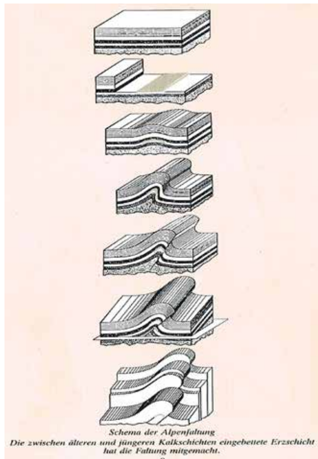
Schema der Alpenfaltung.
